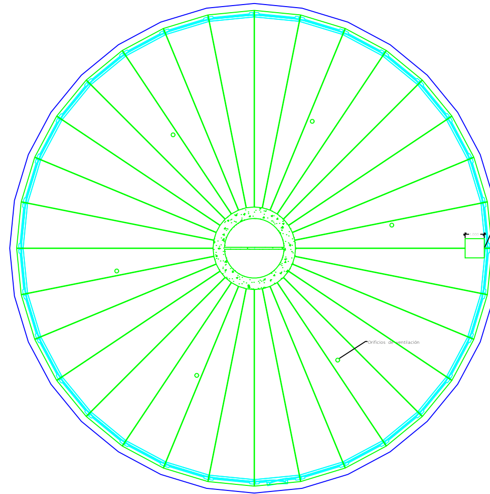
PLANTA DE CUBIERTA
