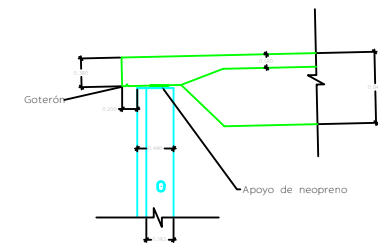
DETALLE 4 E: 1/50
