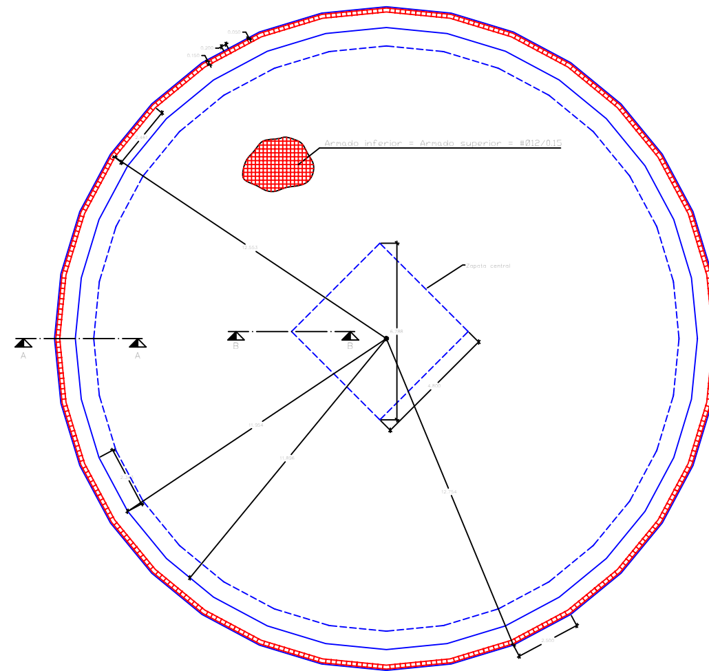
PLANTA DE SOLERA
