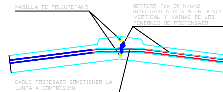
DETALLE 3 E: 1/20
