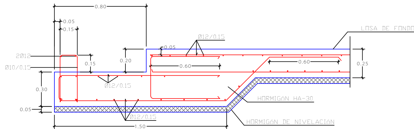
SECCIÓN A - A E: 1/20
