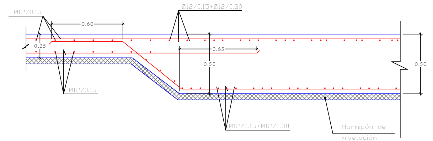
SECCIÓN B - B E: 1/20
